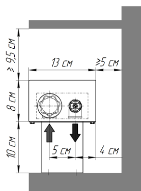
Исполнение "нв" (нерегулируемая высота)
