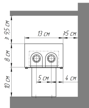
Исполнение "нв" (нерегулируемая высота)
