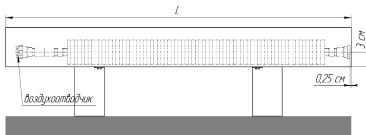
Вид для исполнения "нв" (нерегулируемая высота)
