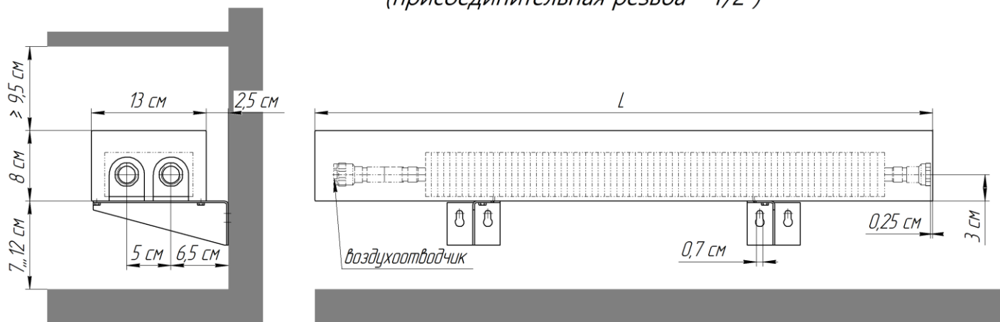
Настенный конвектор "Эlegant - мини 130x80-1то бок Стен прав" с правосторонним боковым присоединением (левостороннее - зеркально) (присоединительная резьба - 1/2")
