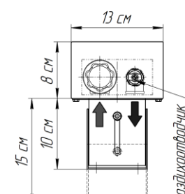
Исполнение "рв" (регулируемая высота)
