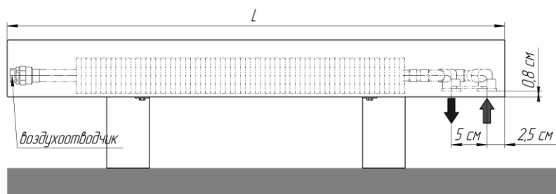
Вид для исполнения "нв" (нерегулируемая высота)
