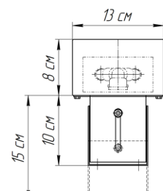
Исполнение "рв" (регулируемая высота)
