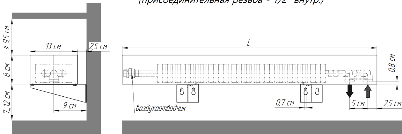
Настенный конвектор "Эlegant - мини 130x80-1то Стен прав" с правосторонним нижним подключением (левостороннее - зеркально) (присоединительная резьба - 1/2" внутр.)
