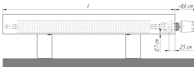
Вид для исполнения "нв" (нерегулируемая высота)
