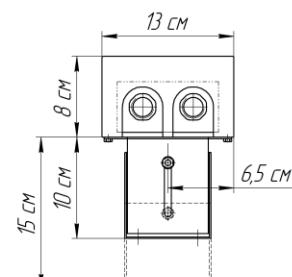
Исполнение "рв" (регулируемая высота)
